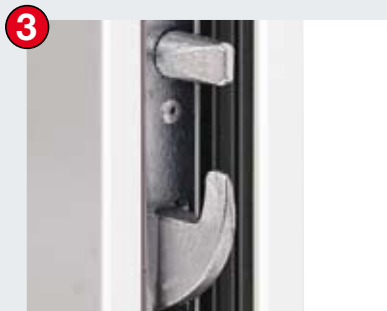
3 Otočná závera s pojistným čepem
